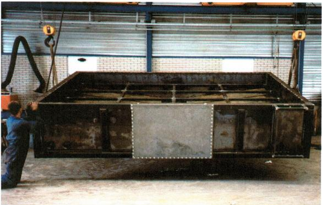
Vloeistofdichte stalen bak ten behoeve van lasersnijwerk.
